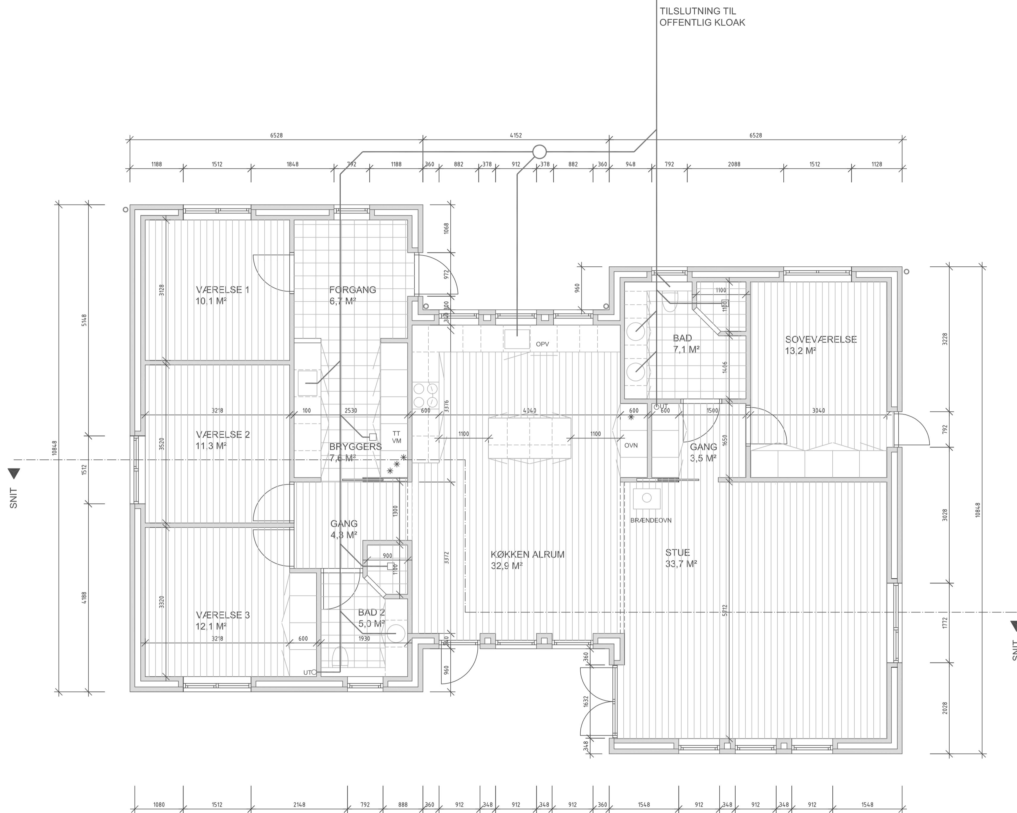
PLAN 1:50
